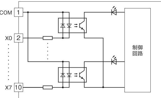
■入力回路
