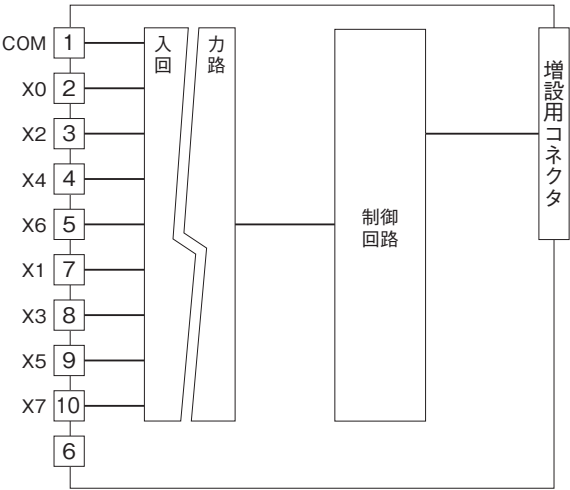
■入力回路
