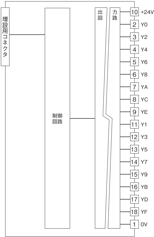
■出力回路
