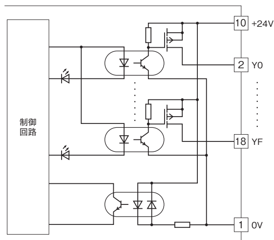
■出力回路
