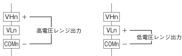
■出力部接続例
