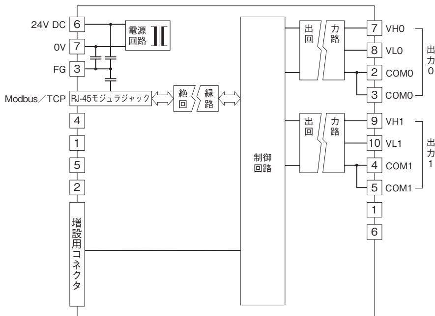
■出力部接続例
