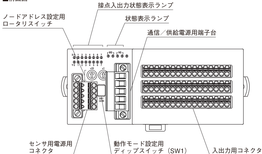
■前面図
