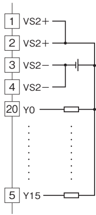
■出力部接続例
