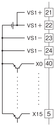
■入力部接続例
