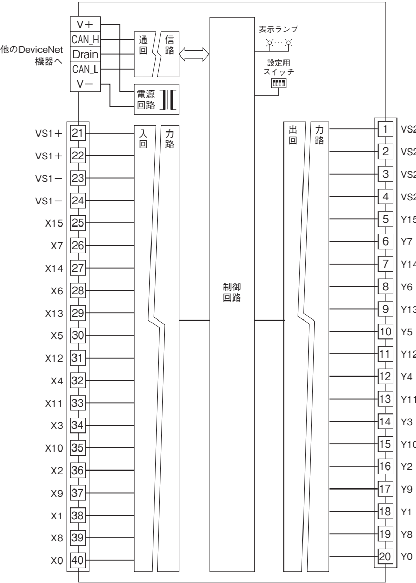
■入力回路
