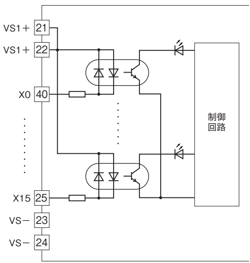
■出力回路
