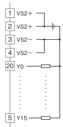
■出力部接続例
