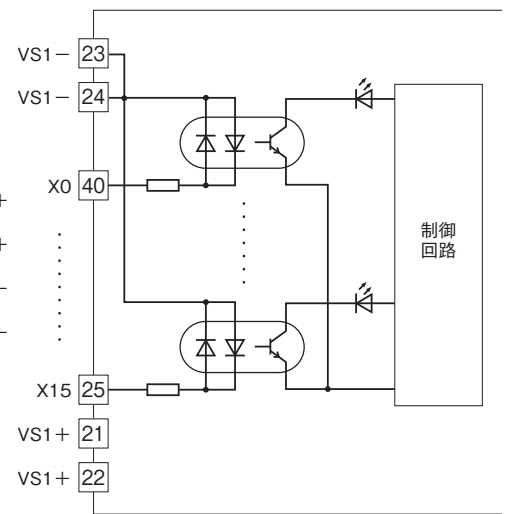
■出力回路
