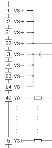
■出力部接続例
