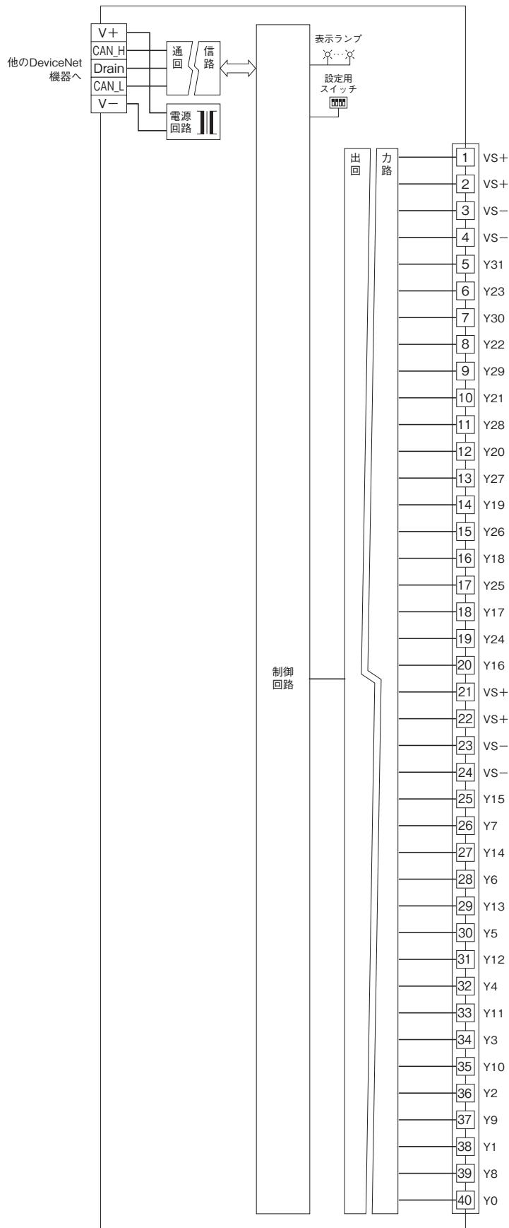
■出力回路
