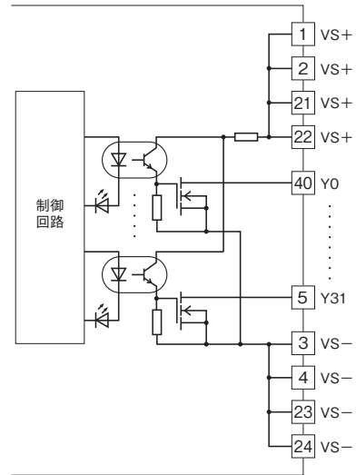
■出力回路
