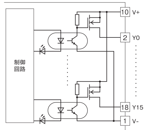
■出力回路
