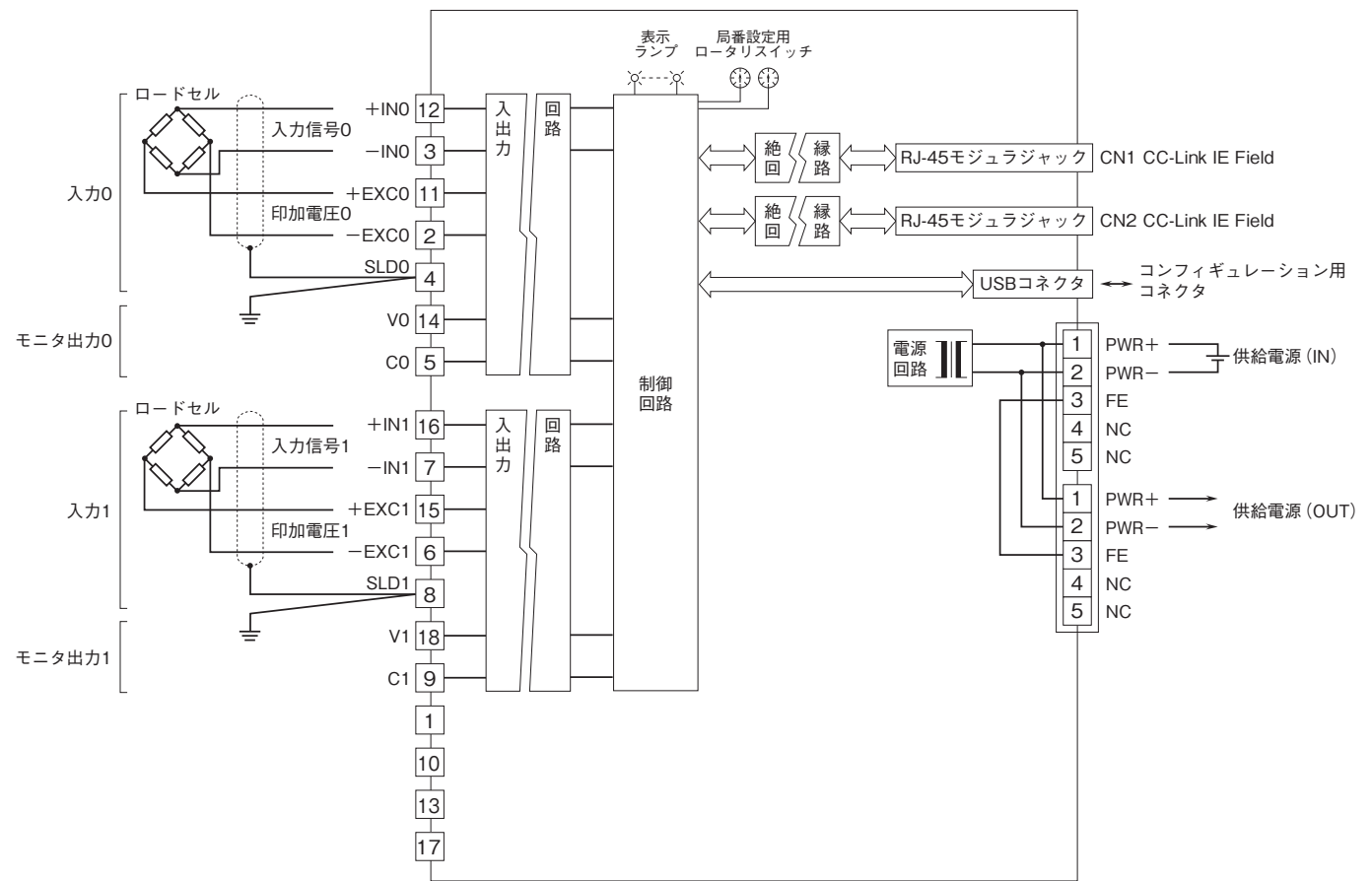
CC-Link IE Field ネットワーク用 RJ-45 モジュラジャック のCN1とCN2は、配線の接続順序に制約はありません。
