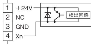
■2線式センサの場合
