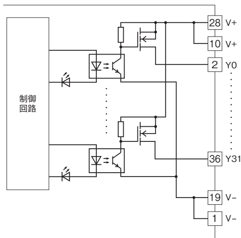
■出力回路
