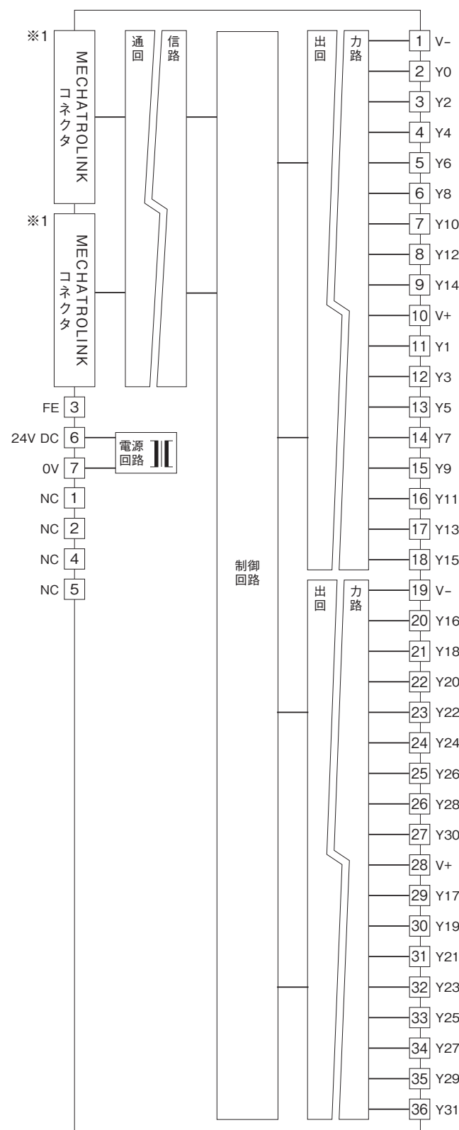
■出力回路
