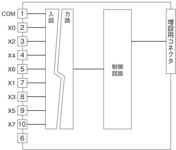
■入力回路
