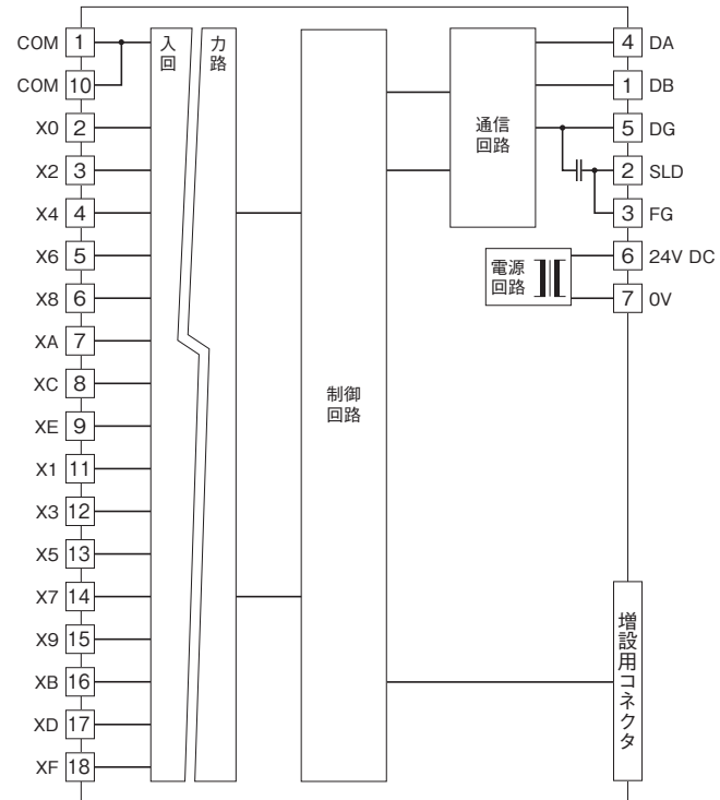
■入力回路
