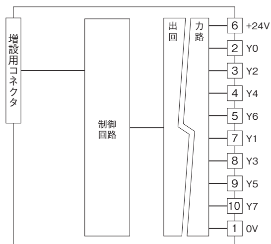
■出力回路
