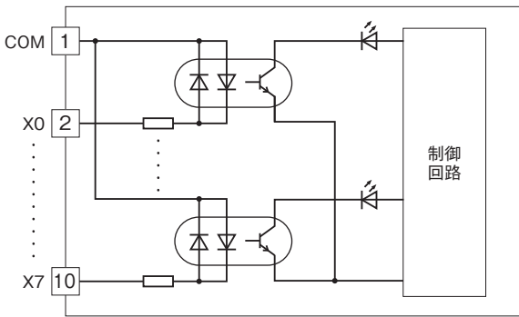
■入力回路
