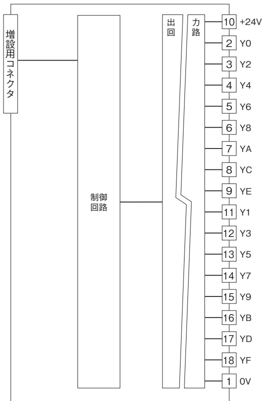
■出力回路
