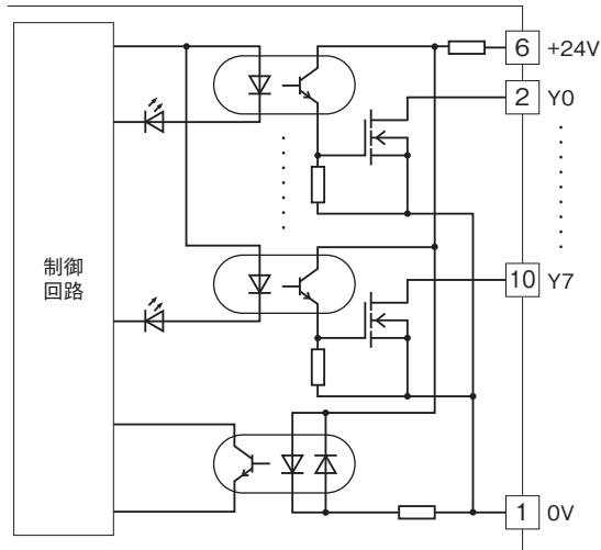
■出力回路
