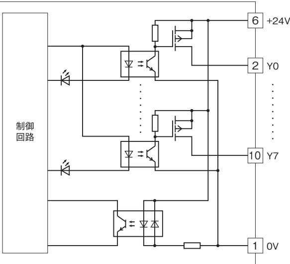
■出力回路
