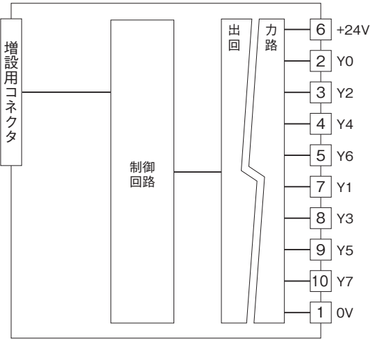
■出力回路
