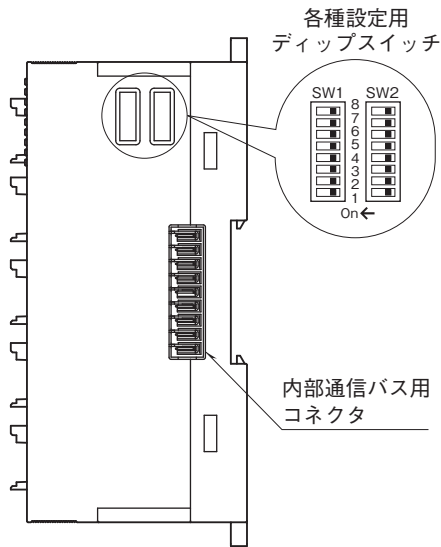
●左側面図
