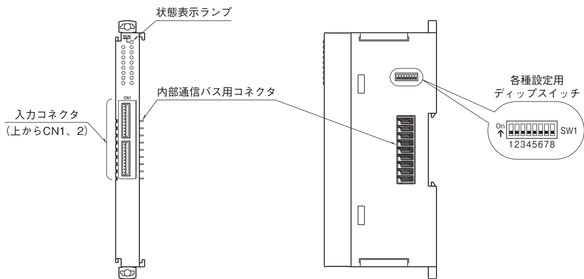
■前面図
