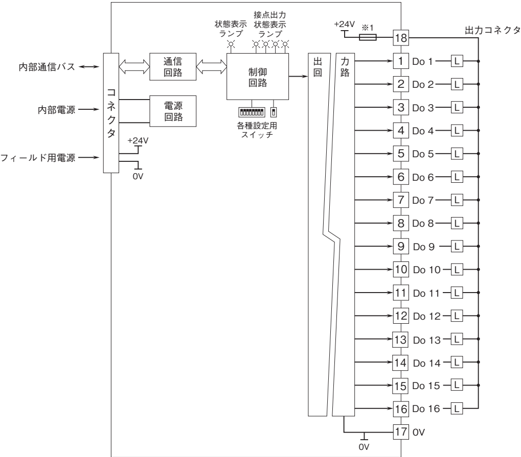
■出力回路
