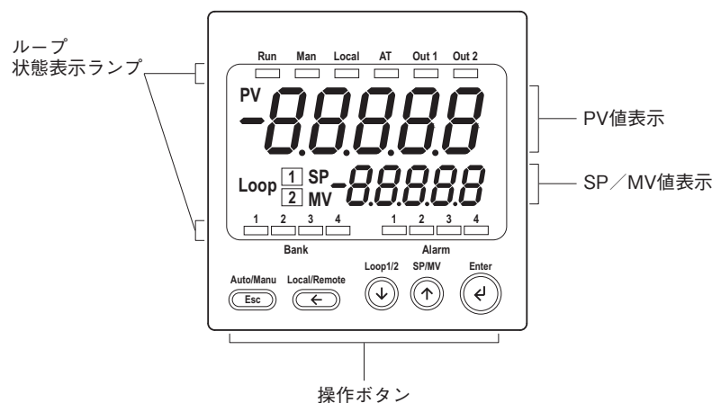
■前面図
