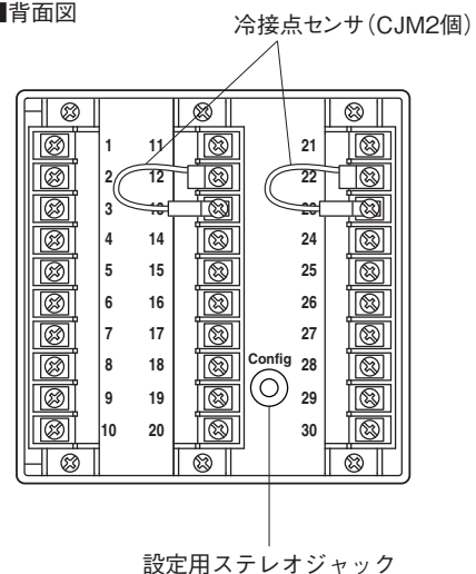
■背面図
