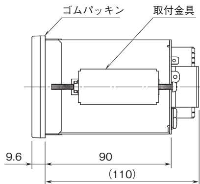
■側面図
