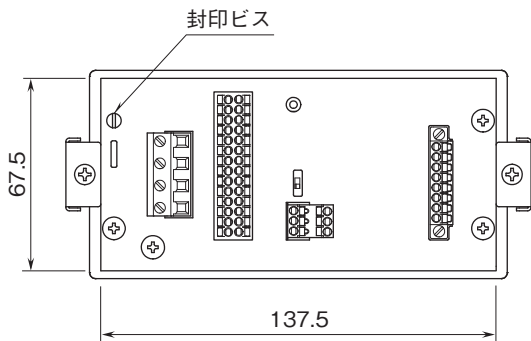
■背面図
