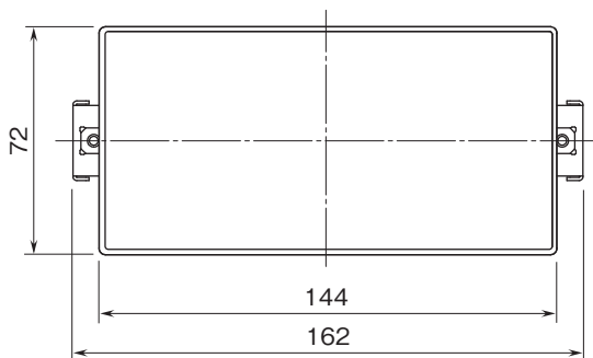
■背面図
