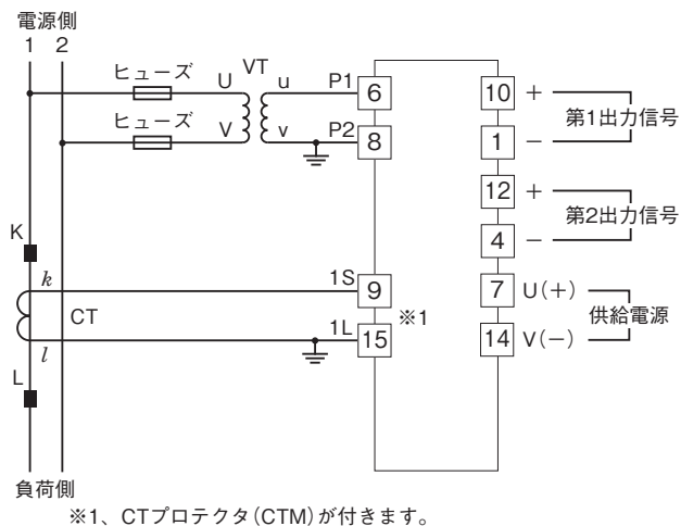
単相2線式
