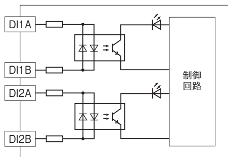
■入力回路
