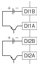
PNP接続
