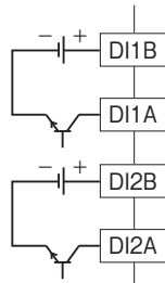
NPN接続
