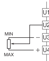
●ポテンショメータ
