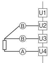
●測温抵抗体および抵抗器 (3線式)
