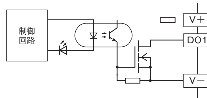
●出力部接続例
