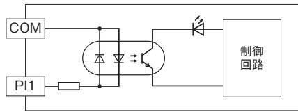
■パルス入力回路
