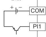
■ユニバーサル入力の接続方法
