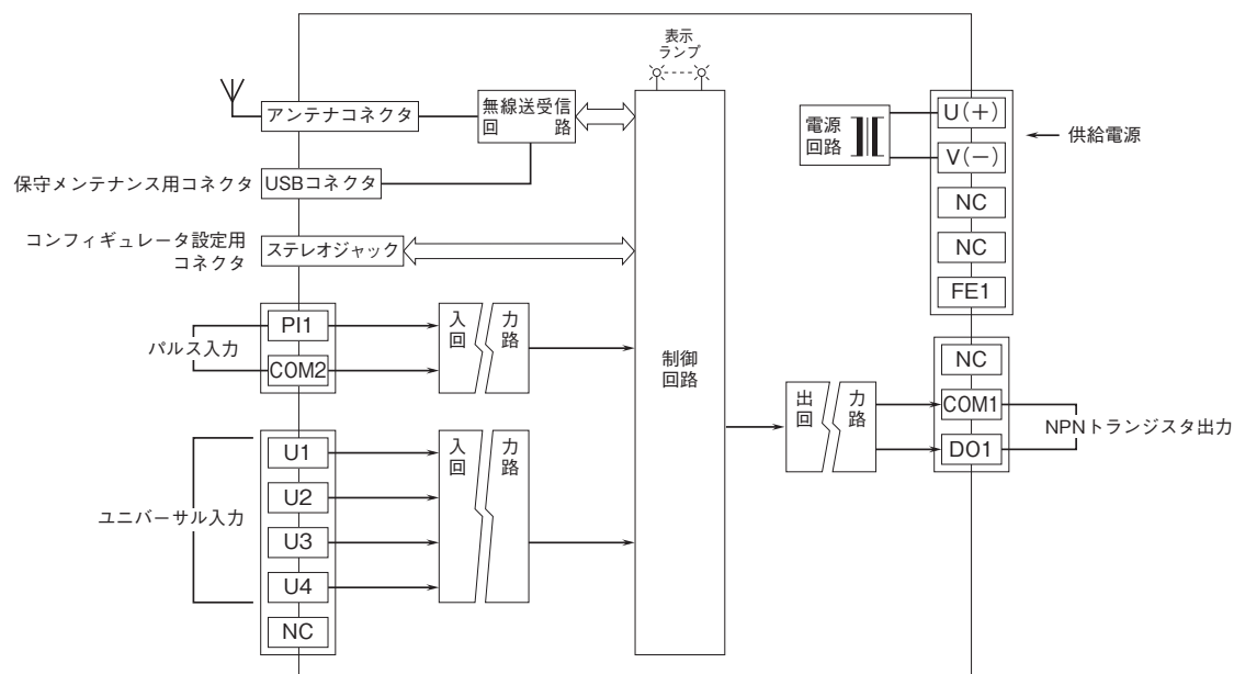
■パルス入力回路
