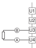
●測温抵抗体および抵抗器 (2線式)
