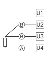
●測温抵抗体および抵抗器 (3線式)
