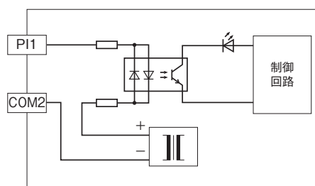
●入力部接続例
