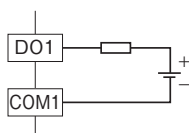
●出力部接続例
