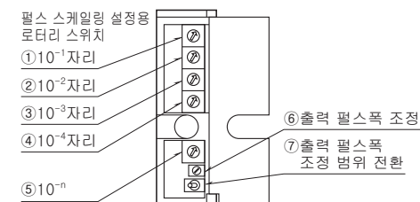
■전면도 (전면 커버가 열린 상태)
