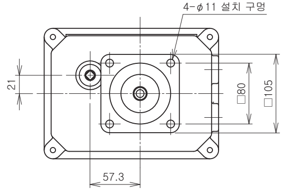
요크 장착부 치수도
