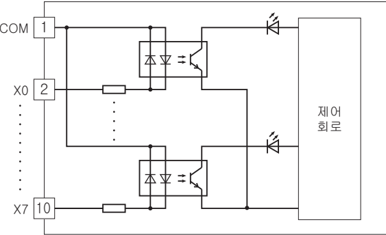
■입력 회로
