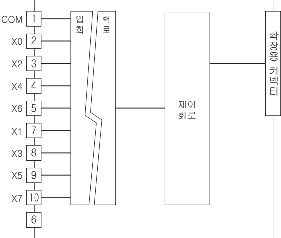
■입력 회로
