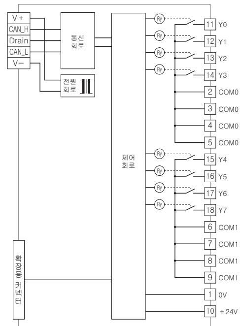
■출력 부분 연결 예
