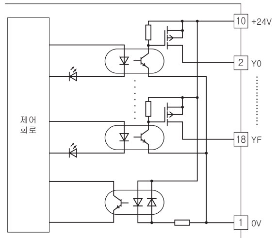
■출력 부분 연결 예
