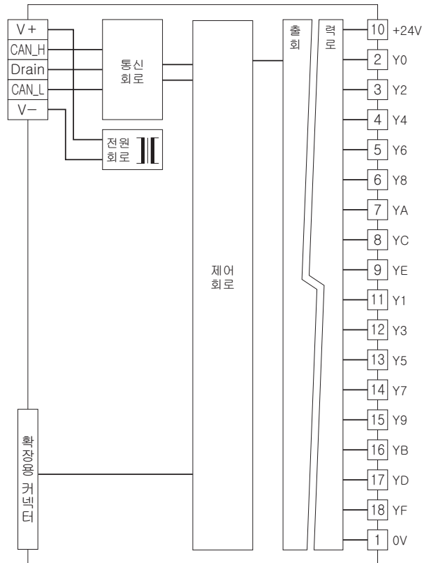
■출력 회로
