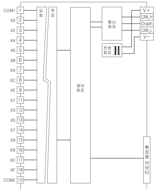
■입력 회로
