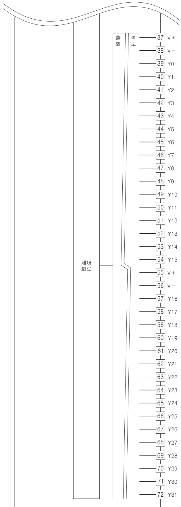
■ 출력 회로
