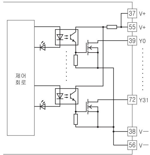
■ 출력 회로
