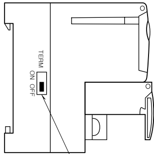
종단 저항 설정용 스위치 ※3
