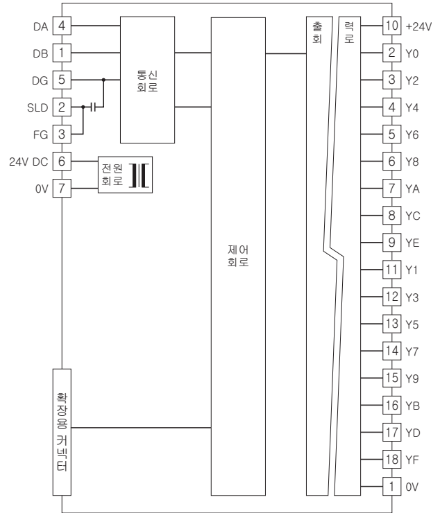
■출력 회로
