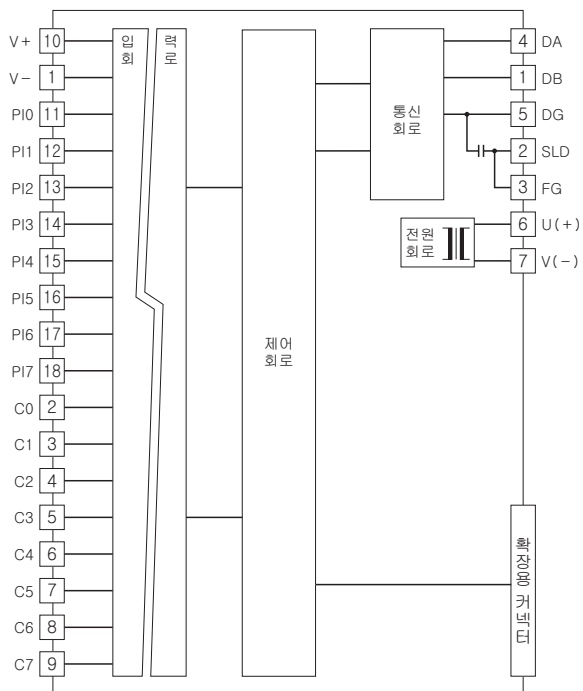
■입력 회로
