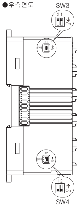
●우측면도
